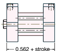
0.875 + carrera Cilindro de doble efecto Vástago sencillo AF-xDR-12x
